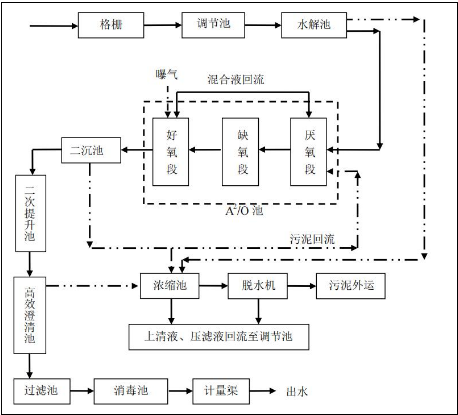
图3.5-1 污水处理工艺流程图
